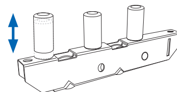
Tándem regulable ( Para hoja Puerta) con chimeneas de apoyo en el refuerzo 140 Kg. Peso máximo de hoja. K-GT-1004-28,8 ( 28,8 mm de altura de chimenea ) K-GT-1004-23,3 ( 23,3 mm de altura de chimenea )
