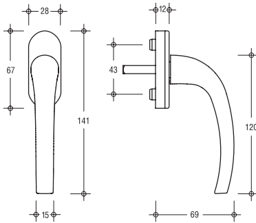
Manilla MODENA 6-31977-33-0-* (Acabados 11,7,5,6 y 3) 6-31977-38-0-* (Acabados 11,7 y 5) * Colores: 7;Blanco, 5; Marrón ,6; Negro 3; Dorado F3 ó 11 Plata.
