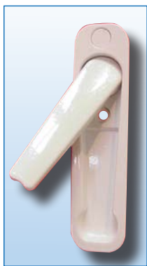
Cierre embutido Referencia : E-35611-08-3- Colores : 7=Blanco; 5= Marrón Profundidad 11 mm.
