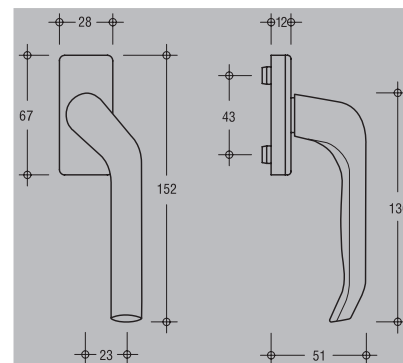
▼ Manilla ADAGIO Acodada sin cuadradillo 6-31221-00-0-* Mano Dcha 6-31323-00-0-* Mano Izda * 7 Blanco ; 5 Marrón
