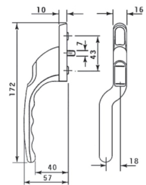
Manilla Acodada Izquierda Ref. 0141-01L-BLANCO 0141-01L-NEGRO
