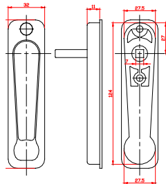
Cierre embutido Referencia : E-35611-08-3- Colores : 7=Blanco; 5= Marrón Profundidad 11 mm.
