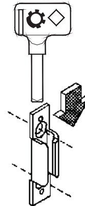
Cerradero E-13880-00-0-1 ( para colgar la manilla de quita y pon)
