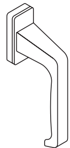
DIRIGENT-F/H de cuello alto, sin cuadradillo 6-28102-00-0-
