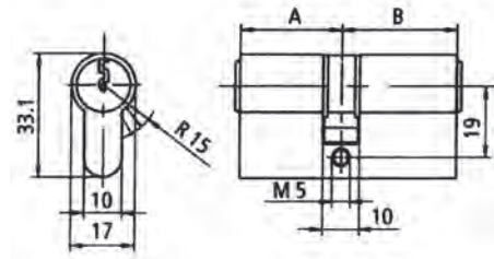
CILINDROS SERIE 50
