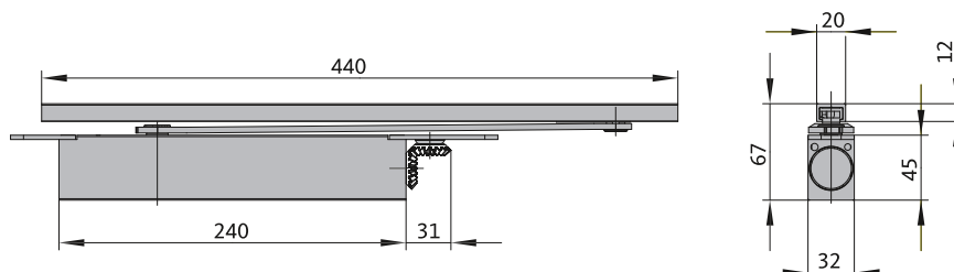
Cierrapuertas oculto VTS 735 con guía deslizante estándar
