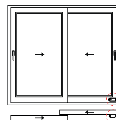
Bolsa de tope 90 Blanco: K-12024-00-0-7 Negro: K-12024-00-0-6
