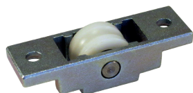
Rueda Fija ventana 60 Kg. Peso máximo de hoja. P-76433-12-0-1
