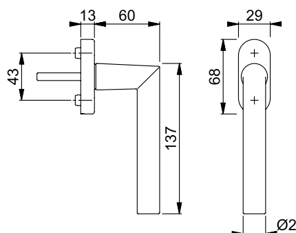
Manilla AMSTERDAN INOX MATE cuadradillo 7x40 3846301-INOX
