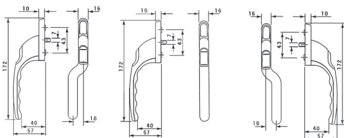
Manilla Acodada Izquierda Ref. 0141-01L-BLANCO 0141-01L-NEGRO
