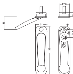
Cierre embutido Referencia : E-35611-08-3-* Colores : 7=Blanco; 5= Marrón Profundidad 11 mm.
