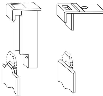
Corte de forma con presna-troquel
